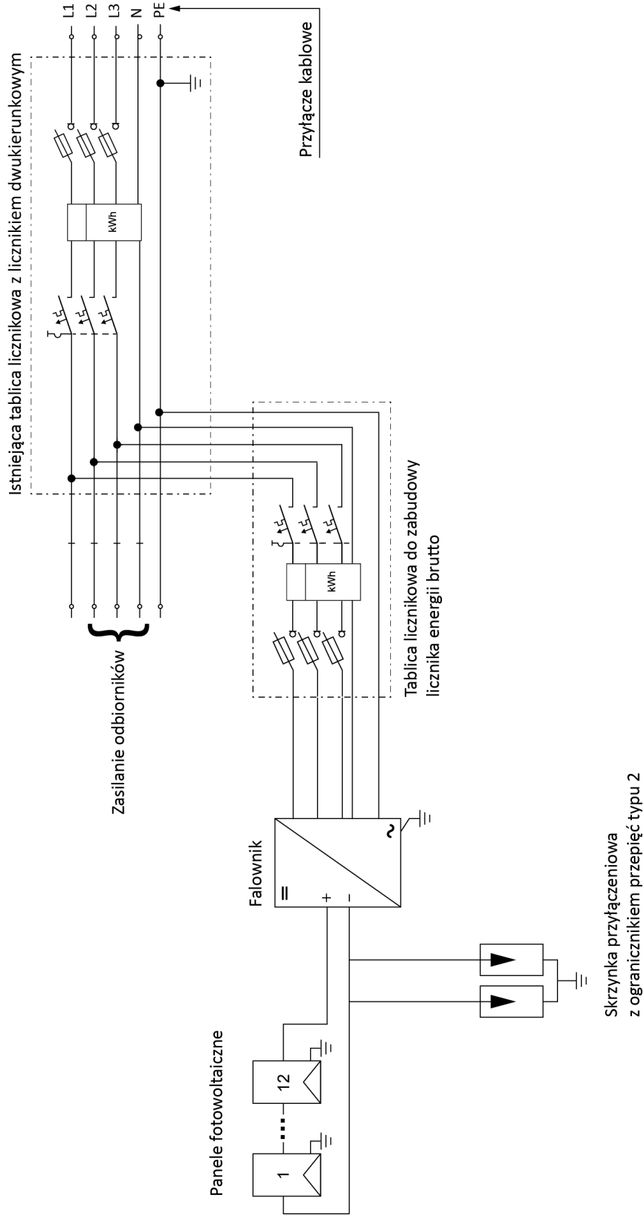
Schemat ideowy instalacji fotowoltaicznej
